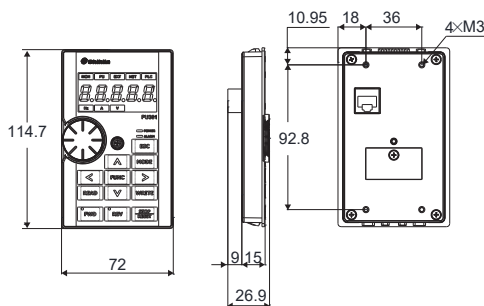
外型尺寸圖
