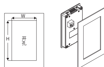
卡扣安裝開孔尺寸圖
